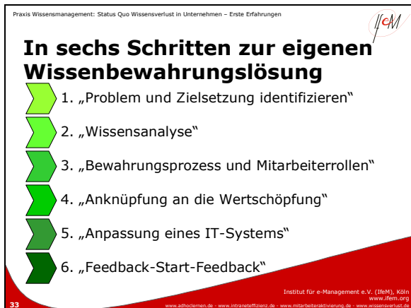
Abbildung 2: Ifem - Vorgehensmodell
