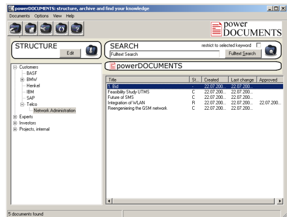
Abbildung 1: powerDOCUMENTS - Hauptfenster
